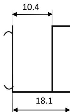
THANH CHẶN LƯNG TỦ (DÀI 6000)
