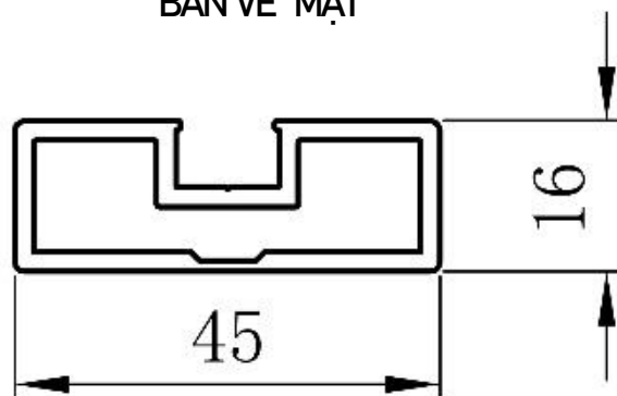
KHUNG CÁNH HỆ VUÔNG
