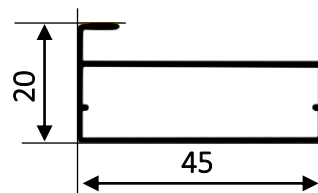
THANH KHUNG MSP 1: BEN-002 MSP 2: PH-3158 Kích thước : 20 x 45
