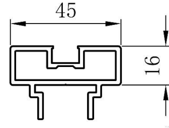
THANH NGANG LÙA TRÊN DƯỚI
