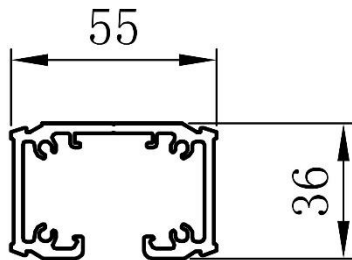
RAY ĐƠN ÂM TƯỜNG ( TRẦN )
