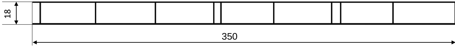
TẤM NHÔM CHO TỦ BẾP TRÊN (18 x 350 x 6000)
