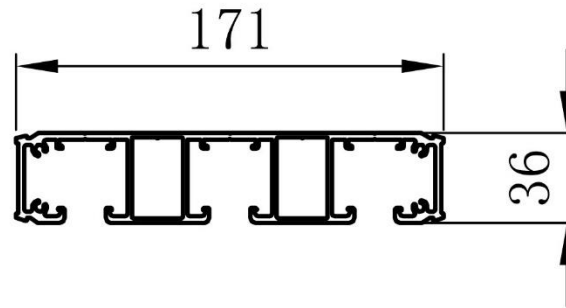
RAY 3 ÂM TƯỜNG ( TRẦN )
