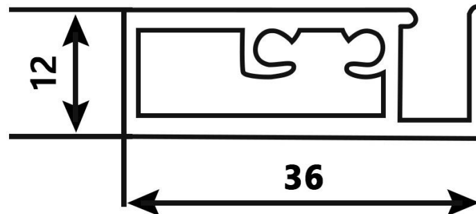
KHUNG NHÔM ĐỂ KHAY RƯỢU
