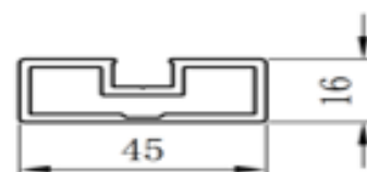
KHUNG CÁNH HỆ VUÔNG
