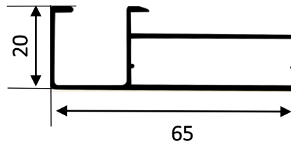
TAY NẮM ÂM MSP 1: BEN-003 MSP 2: PH-3157 Kích thước : 20 x 65
