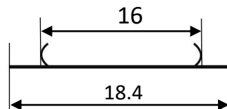
THANH NẸP CẠNH (DÀI 6000)
