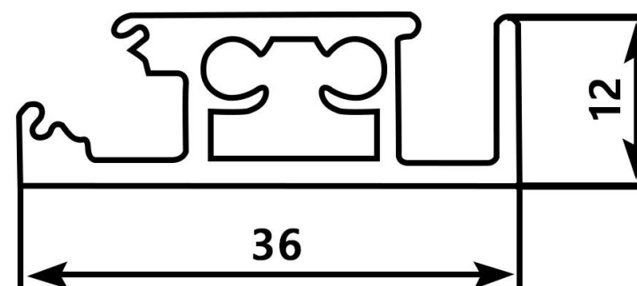
MẶT CẮT KHUNG NHÔM TÍCH HỢP ĐÈN LED
