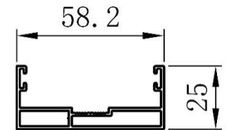
CÂY KHUNG BAO ĐỨNG
