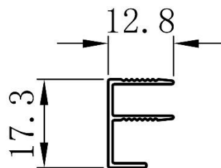
KHUNG BAO NHỎ
