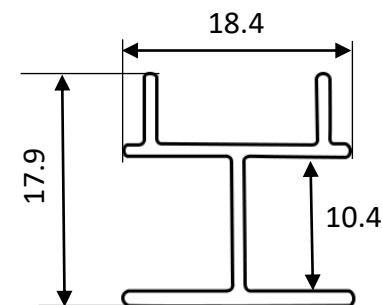
NẸP NỐI HẬU (DÀI 4000)
