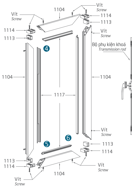
Chi tiết ráp khung cánh Leaf frame details
