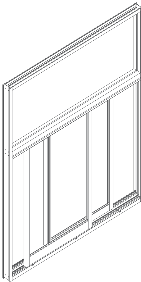
Lắp ráp hoàn thiện Complete assembly diagram
