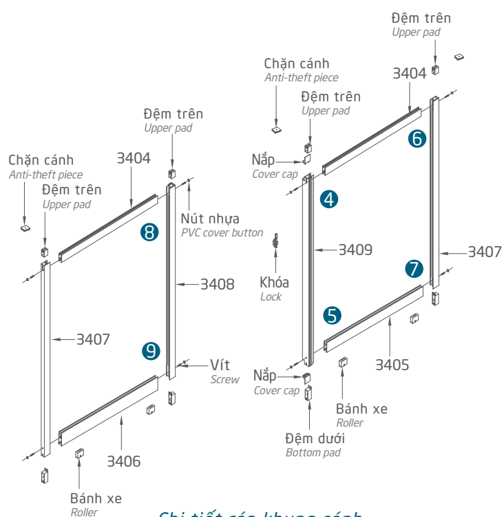
Chi tiết ráp khung cánh Leaf frame details
