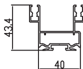
Khung bao cửa lùa
