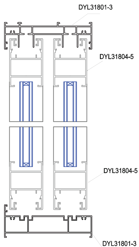
MẶT CẮT 1-1
