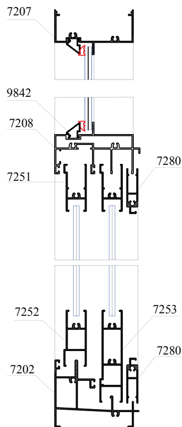
MẶT CẮT 1-1
