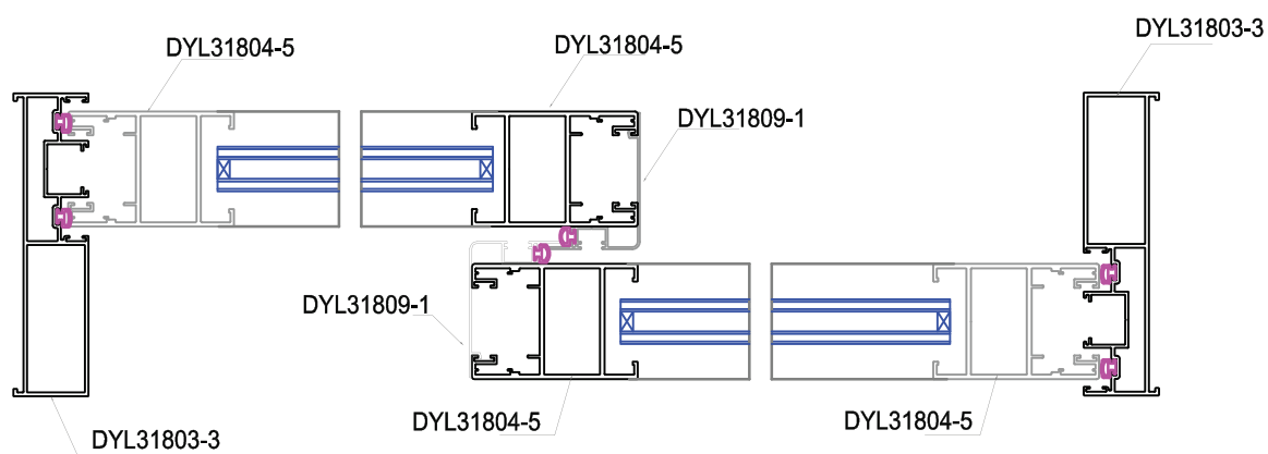
MẶT CẮT 2-2
