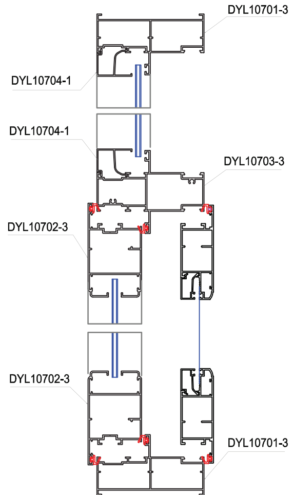
MẶT CẮT 1-1
