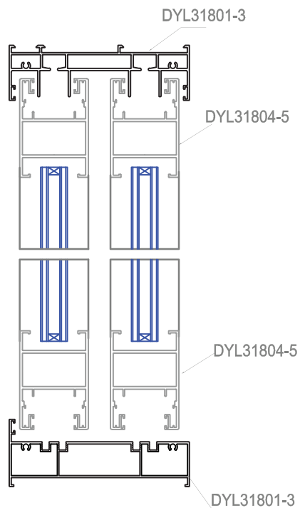
MẶT CẮT 1-1
