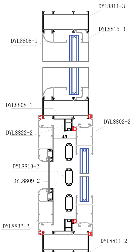
MẶT CẮT 1-2-3
