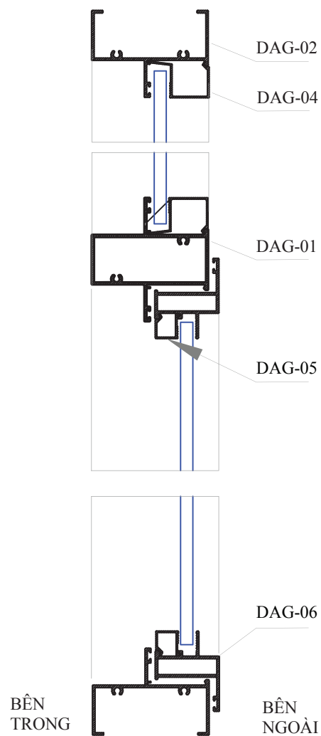
MẶT CẮT 1-1
