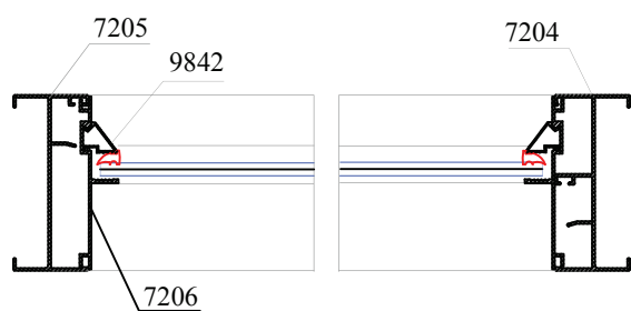
MẶT CẮT 3-3
