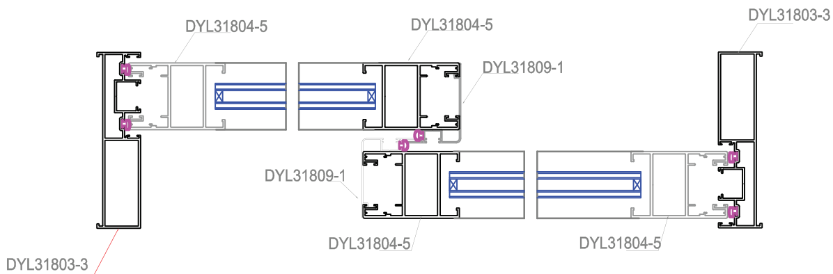
MẶT CẮT 2-2
