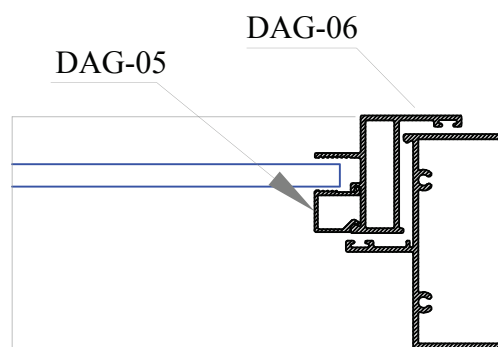
MẶT CẮT 2-2
