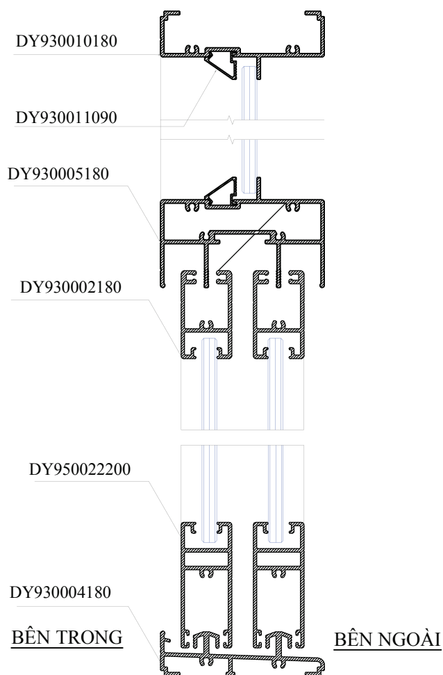
MẶT CẮT 1-1
