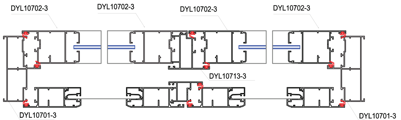
MẶT CẮT 2-2
