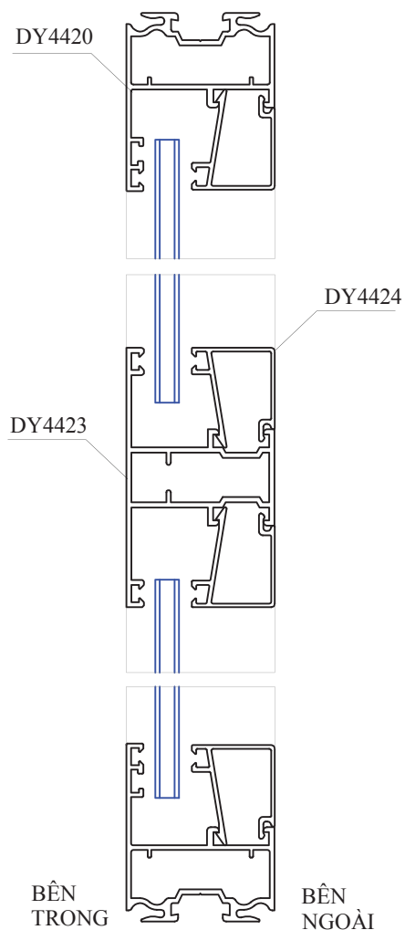
MẶT CẮT 1-1
