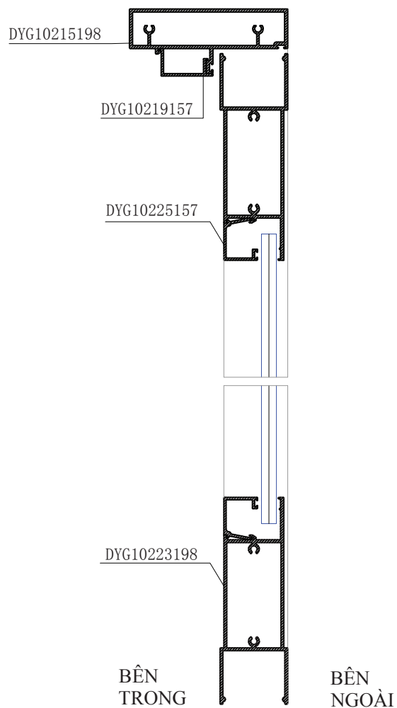
MẶT CẮT 1-1
