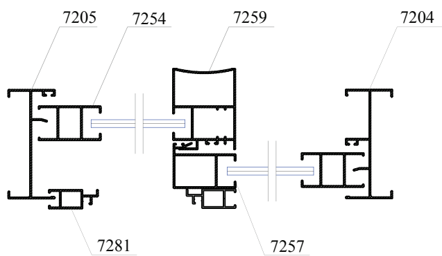
MẶT CẮT 2-2
