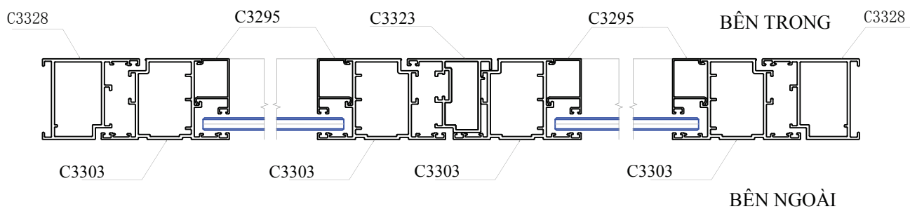
MẶT CẮT 2-2
