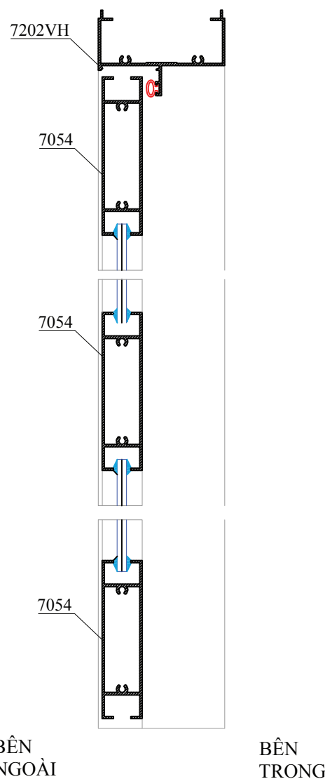
MẶT CẮT 1-1
