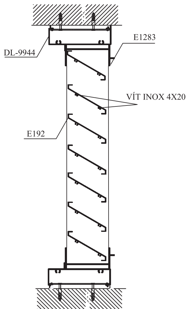
MẶT CẮT 1-1
