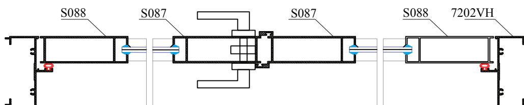
MẶT CẮT 2-2
