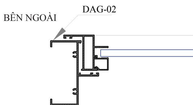
MẶT CẮT 2-2
