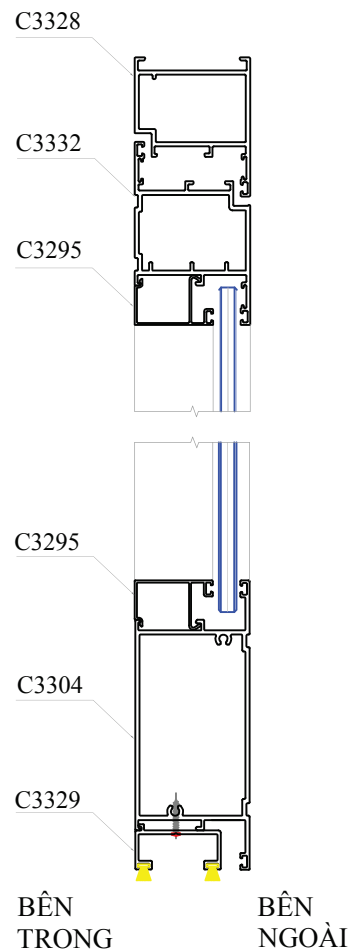
MẶT CẮT 1-1
