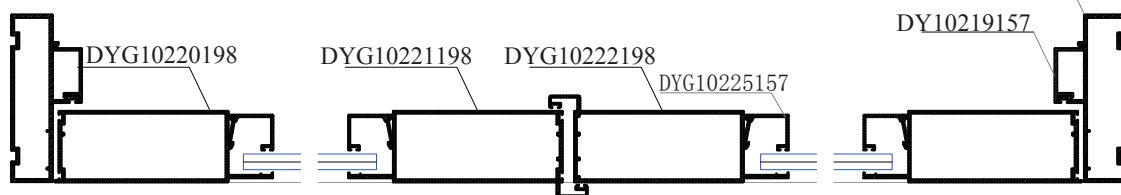
MẶT CẮT 2-2
