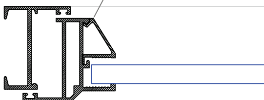
MẶT CẮT 2-2
