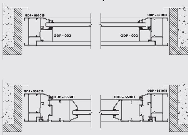
MẶT CẮT 2-2
