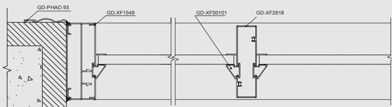
MẶT CẮT 3-3
