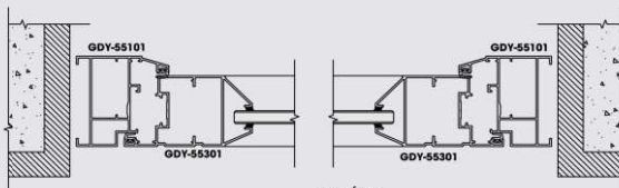
MẶT CẮT 3-3
