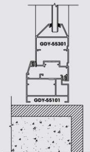
MẶT CẮT 1-1
