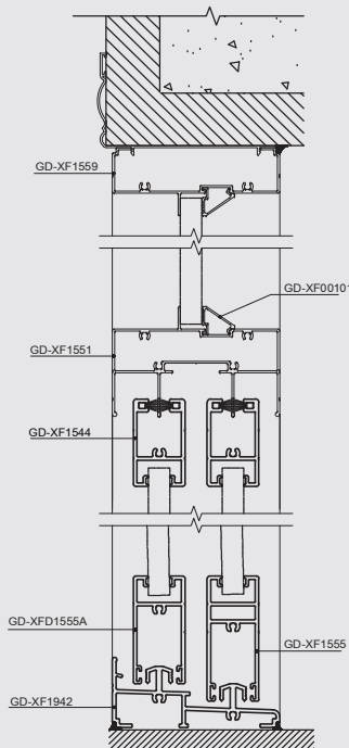
MẶT CẮT 1-1
