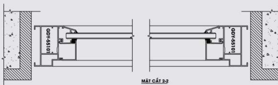
MẶT CẮT 2-2
