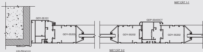
MAT CẮT 2-2
