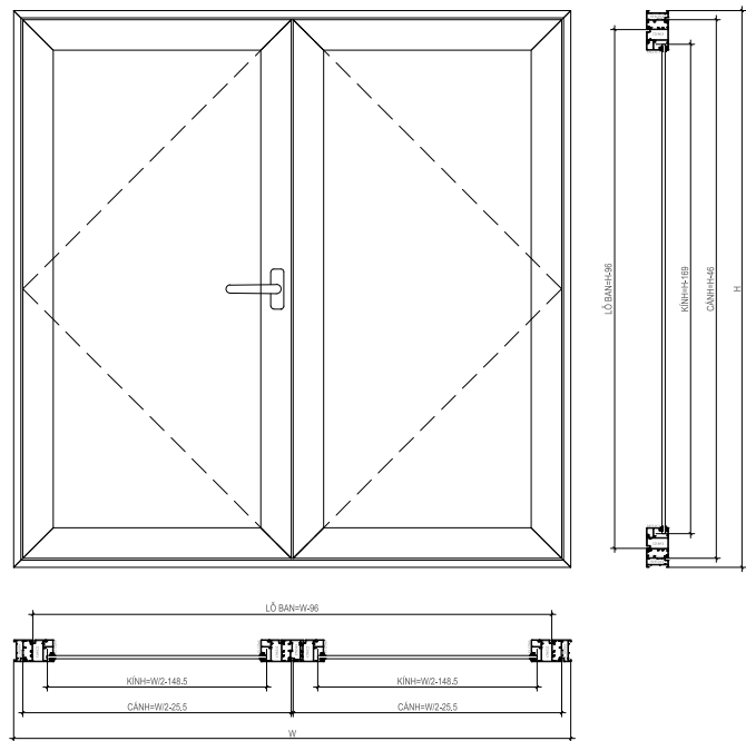
CỬA SỔ 2 CÁCH MỞ NGOÀI
