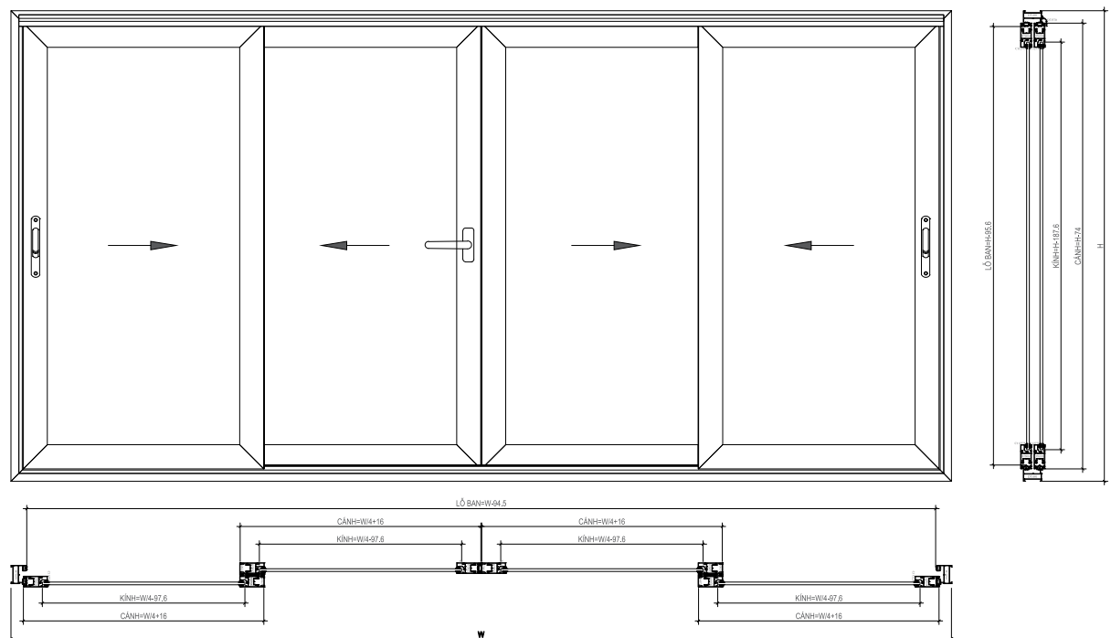
CỬA SỔ 4 CÁCH MỞ LÙA
