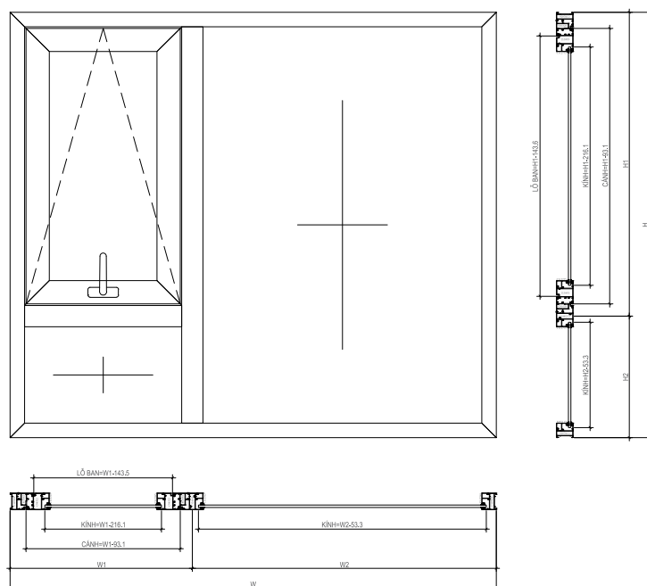
CỬA SỔ 1 CÁNH MỞ NGOÀI + VÁCH KÍNH
