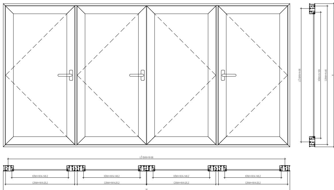
CỬA SỔ 4 CÁCH MỞ NGOÀI
