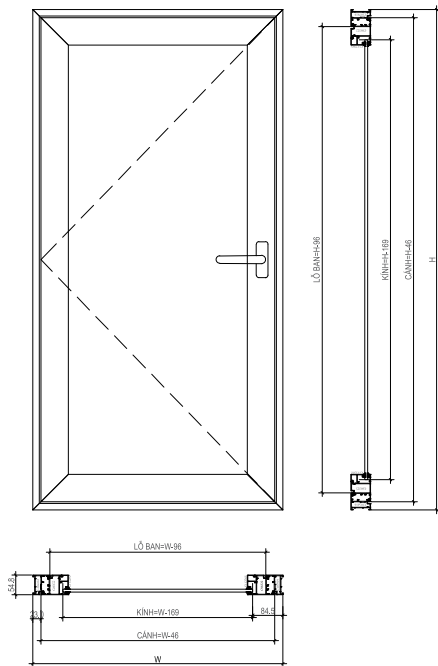
CỬA SỔ 1 CÁCH MỞ NGOÀI
