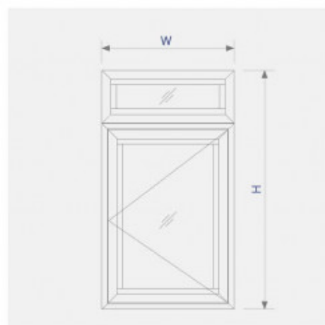
Sơ đồ lắp ráp cửa sổ mở quay 1 cánh hệ XFA1000
