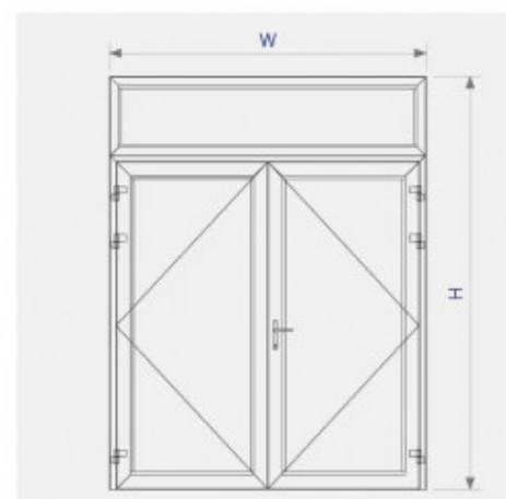
Sơ đồ lắp ráp cửa đi mở quay 2 cánh hệ XFA1000
