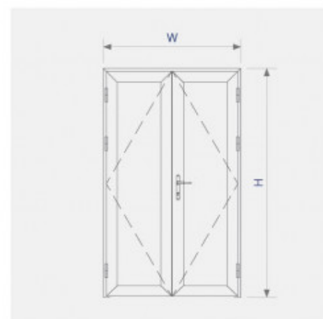
Sơ đồ lắp ráp cửa đi mở quay 2 cánh hệ XFA55
