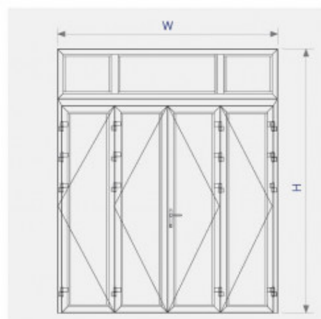
Sơ đồ lắp ráp cửa đi mở quay 4 cánh hệ XFA1000
