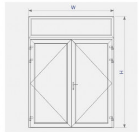
Sơ đồ lắp ráp cửa đi mở quay 2 cánh hệ XFA55
