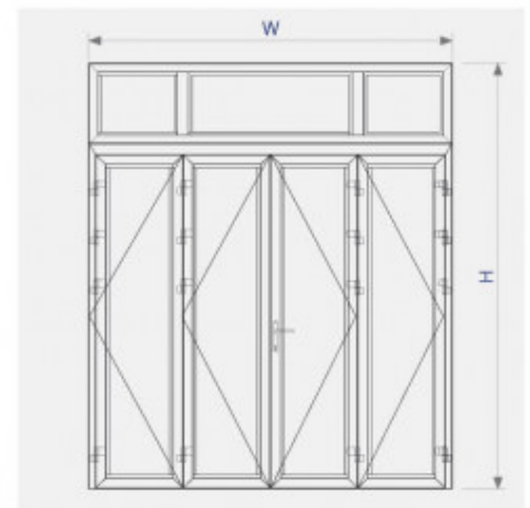
Sơ đồ lắp ráp cửa đi mở quay 4 cánh hệ XFA55
