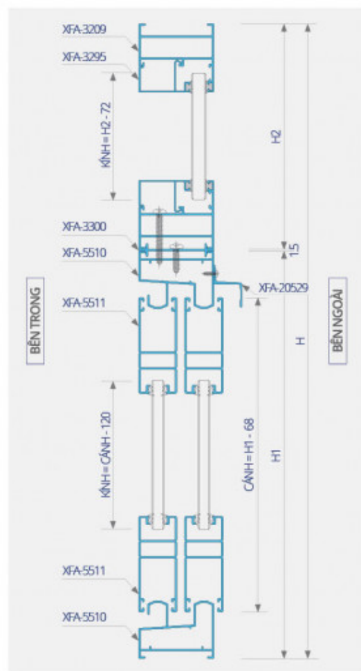
Sơ đồ lắp ráp cửa sổ lùa hệ XFA55
