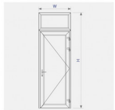
Sơ đồ lắp ráp cửa đi mở quay 1 cánh hệ XFA55
